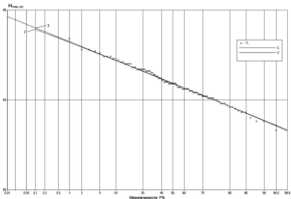
Рис. А.21. Кривая обеспеченности максимальных уровней воды р. Обь — д. Медведово 1 — эмпирические точки, 2 — кривая обеспеченности, рассчитанная по параметрам ряда, 3 — кривая обеспеченности при C_s/C_v=0,01
