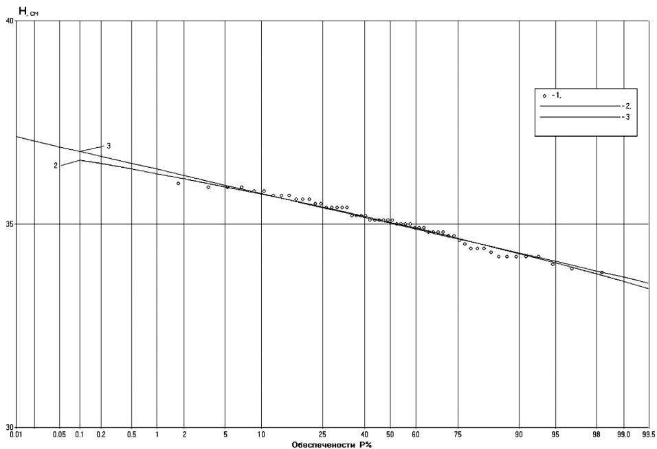
Рис. А.22. Кривая обеспеченности среднегодовых уровней р. Обь — д. Медведово 1 — эмпирические точки, 2 — кривая обеспеченности по параметрам, рассчитанным по ряду, 3 — кривая обеспеченности при C_s/C_v=0,01
