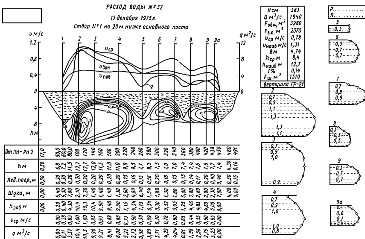
Рис.6.14. Образец графической обработки расхода воды
