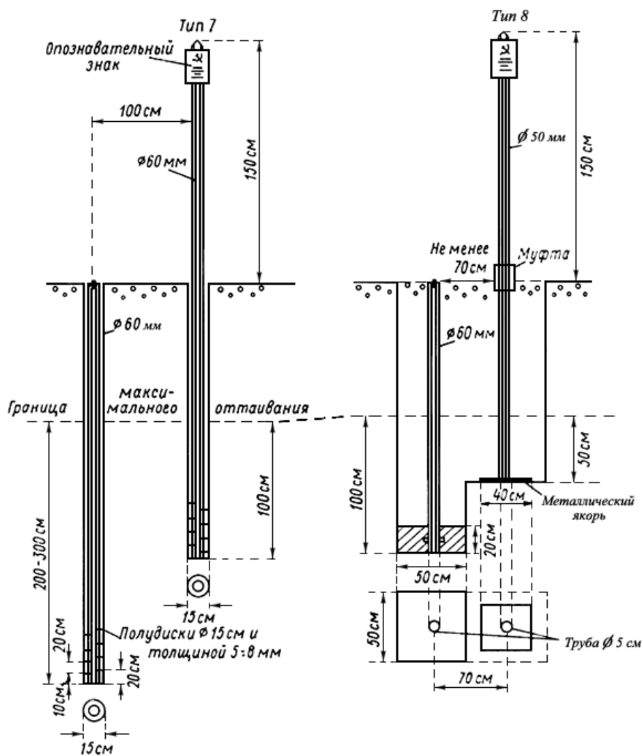
Рис 7. Грунтовые реперы в зоне распространения многолетней мерзлоты
