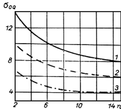
Рис.12.5. Зависимость погрешности ежедневных расходов воды \sigma_{0Q} от частоты измерений ( n - количество измерений в месяц)
