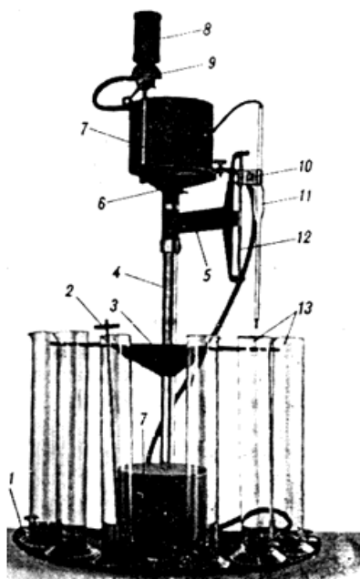
Рис.8.7. Пипеточная установка ПИ-22
