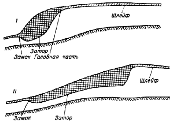
Рис.10.4. Схематические продольные профили заторов льда I - затор с выраженной головной частью; II - затор с равномерным продольным профилем.
