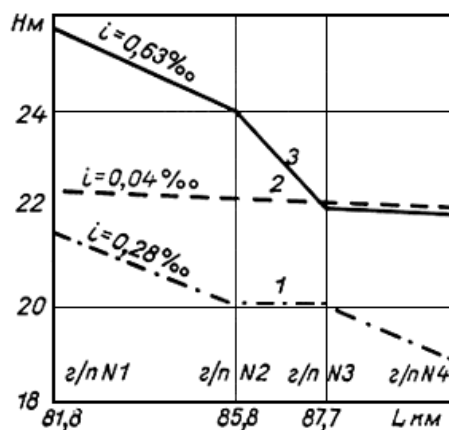
Рис.10.7. Характерные продольные профили водной поверхности на зажорном участке р.Белой
