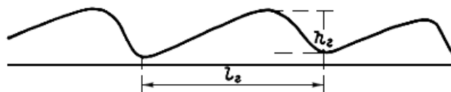
Рис.12.8. Схематический профиль донных гряд
