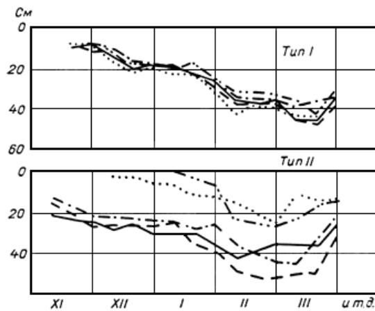
Рис.10.3. Графики нарастания толщины льда на участке реки (по наблюдениям в пяти точках)
