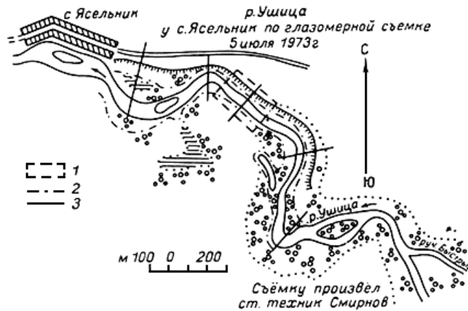
Рис.2.1. План участка реки в районе намечаемого поста, составленный по глазомерной съемке 1 - граница намеченного участка; 2 - урез воды при наивысшем уровне; 3 - профили
