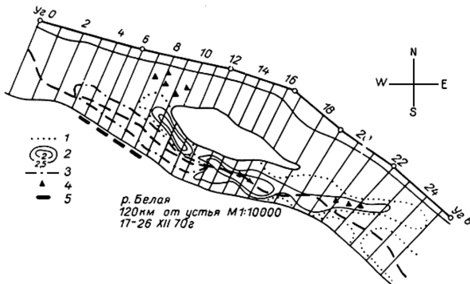
Рис.10.5. Схематический план зажорного участка
