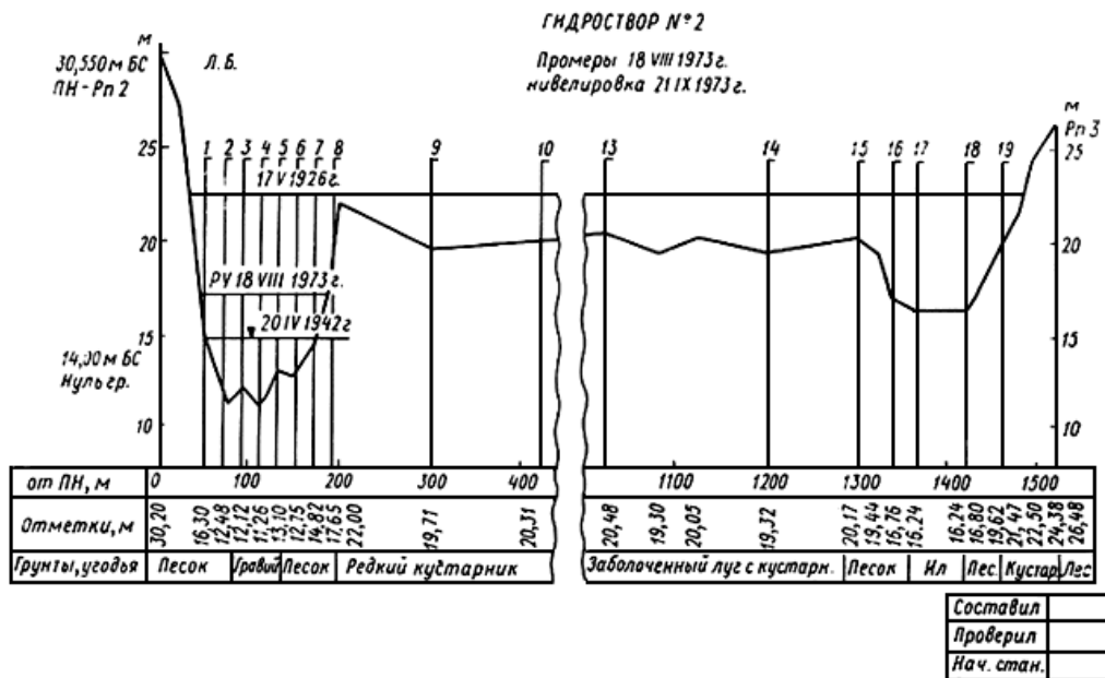
Рис.6.2. Профиль гидрометрического створа
