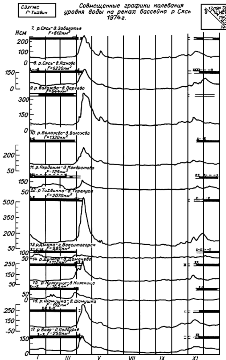
Рис.4.3. Совмещенные графики колебания уровня воды на реках бассейна р.Сясь
