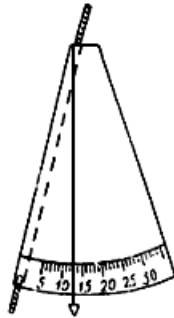
Рис.6.4. Угломер для измерения угла отклонения каната от вертикального положения
