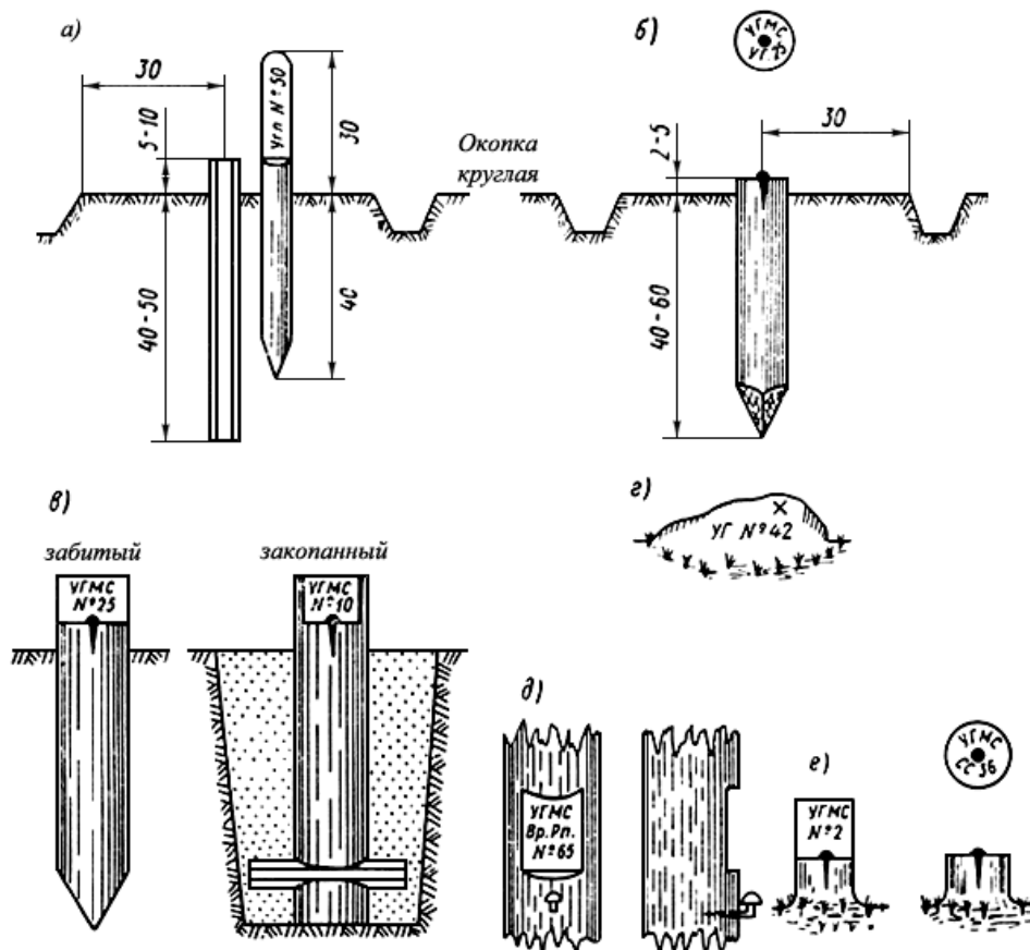
Рис 11. Типы знаков временного закрепления съемочных сетей (плановых и высотных)
