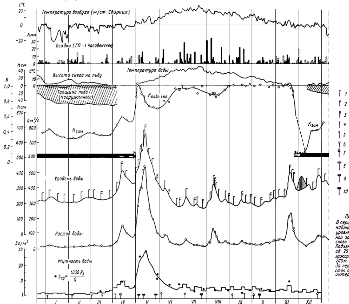
Рис.4.2. Комплексный график результатов гидрометеорологических наблюдений 1 - расход воды; 2 - расход воды и взвешенных наносов; 3 - расход воды, взвешенных и донных наносов; 4 - промер русла; 5 - контрольная нивелировка поста; 6 - съемка течений; 7 - взятие проб воды на химический анализ; 8 - отбор проб на гранулометрический состав взвешенных наносов; 9 - отбор проб на гранулометрический состав донных наносов; 10 - отбор проб на гранулометрический состав взвешенных и донных наносов
