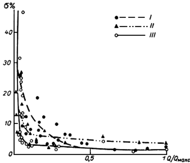
Рис.12.4. График связи среднеквадратической погрешности расхода воды \sigma с относительной величиной расходов воды Q/Q_{\max} . р.Великая - д.Гуйтово. 1971-1972 гг.
