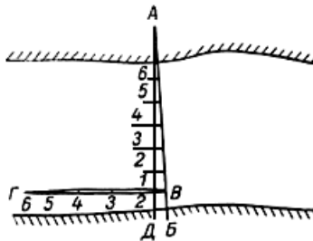
Рис.6.1. Разбивка гидрометрического створа с учетом направления течения
