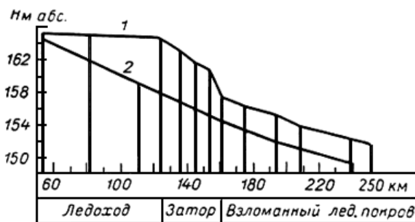
Рис.10.6. Продольный профиль водной поверхности на заторном участке реки 1 - при заторе 27/V 1969 г.; 2 - при открытом русле
