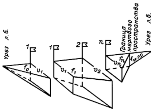
Рис.6.7. Схема к вычислению расхода воды аналитическим методом
