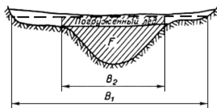
Рис.6.12. Поперечное сечение реки при ледяном покрове, лежащем на берегах
