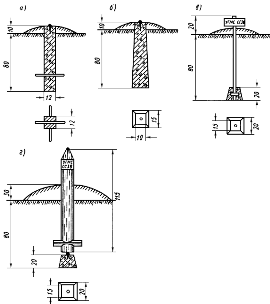
Рис.10. Типы знаков долговременного закрепления съемочных сетей
