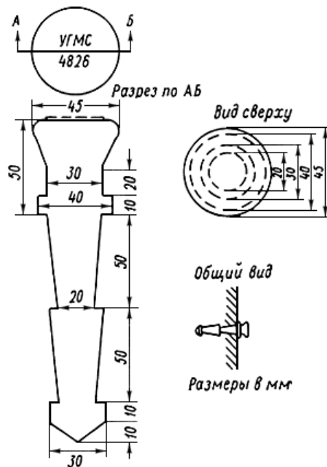
Рис.9. Стенной репер
