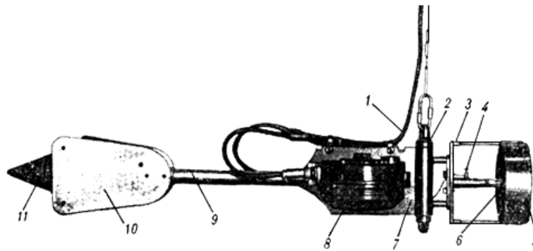
Рис.1. Измеритель течения ГР-42
