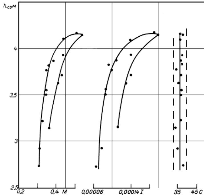
Рис.5.4. Зависимости параметра M = \frac{v_{cp}}{\sqrt{h_{cp}}} , местного уклона водной поверхности I , коэффициента C = \frac{v_{cp}}{\sqrt{h_{cp}I}} от средней глубины (р.Нея - д.Буслаево).
