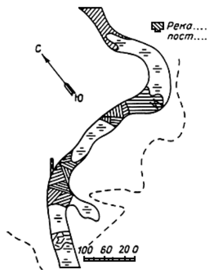
Рис.10.1. Образец картограммы ледовой обстановки на участке реки
