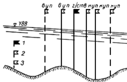
Рис.5.1. Схема расположения створов для измерения уклонов водной поверхности
