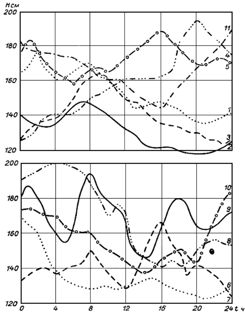
Рис 12.1. Типы (1-11) суточного хода уровня в октябре-ноябре 1966 г. на р.Неве у Горного института
