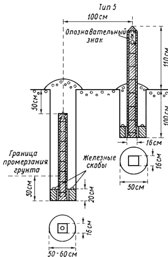
Рис.1. Грунтовый репер нивелирования I, II, III, IV классов для северной зоны сезонного промерзания грунтов
