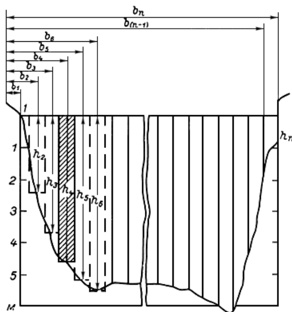
Рис.6.13. Схема к вычислению расхода воды при совмещении промерных и скоростных вертикалей
