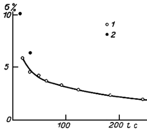
Рис.12.3. Зависимость погрешности в определении средней скорости на вертикали ( \sigma ) при 2-точечном способе измерения от продолжительности выдержки вертушки в точке 1 - по Р.Картеру, 2 - по данным Ботма и Струйка
