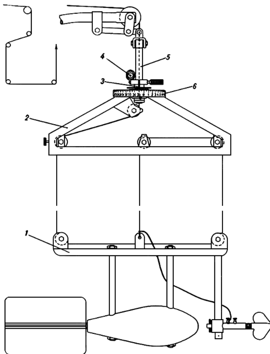
Рис.1. Бифилярный подвес
