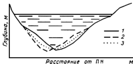
Рис.6.9. Профиль гидрометрического створа по двум ходам
