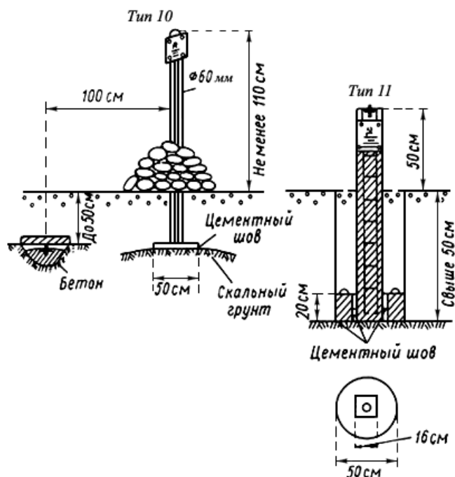
Рис.8. Реперы для скальных грунтов
