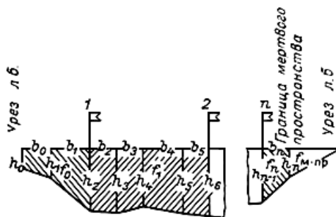
Рис.6.8. Схема к вычислению площади водного сечения
