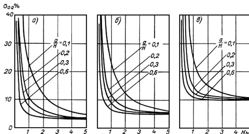
Рис.7.1. Средняя квадратическая погрешность определения расхода воды при незатопленном истечении из-под затворов в зависимости от их относительного открытия \frac{\alpha}{H} ( \alpha - открытие затвора, м; H - действующий напор, м) при различных данных о точности определения коэффициента расхода
