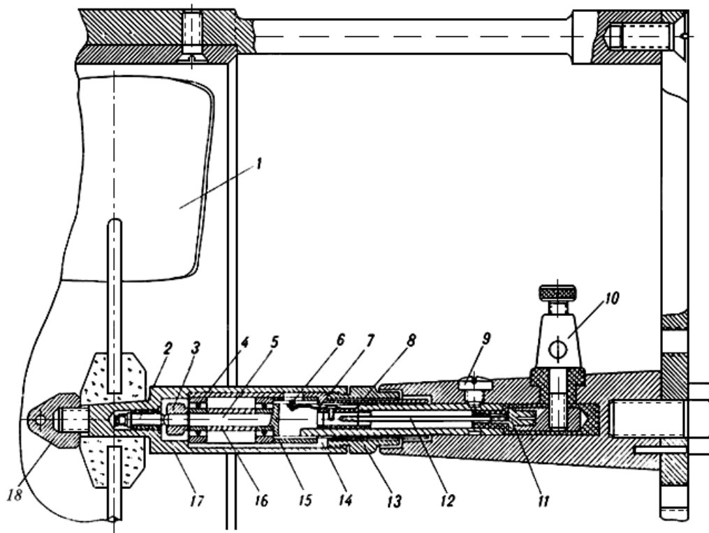
Рис.2. Схема ходовой части вертушки измерителя течения ГР-42
