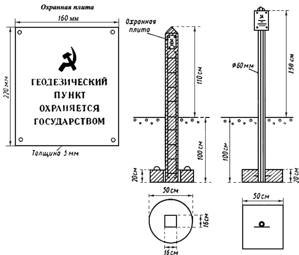
Рис.4. Оповестительные знаки для зоны сезонного промерзания грунта
