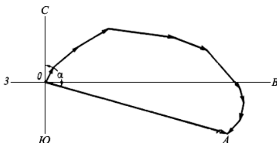
Рис.3. Векториальный график для определения течения геометрическим способом
