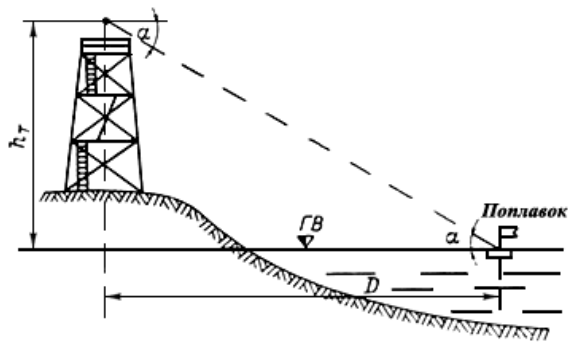
Рис.6.15. Схема засечки поплавков однотоочечным способом
