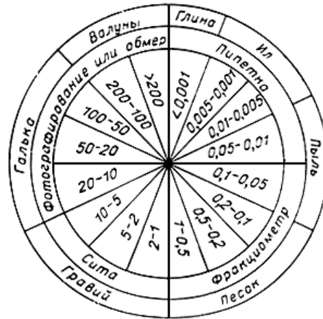
Рис.8.3. Применение методов анализа в зависимости от крупности частиц
