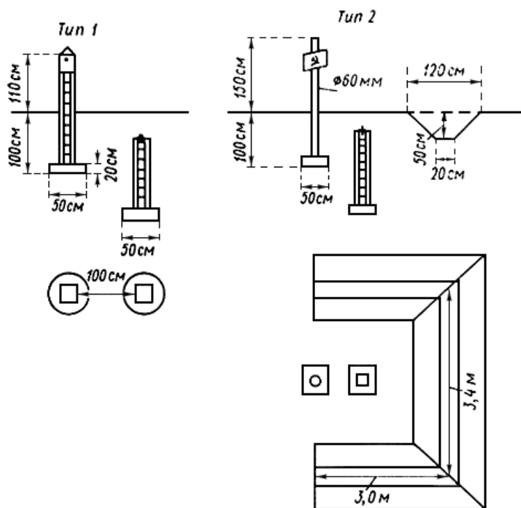
Рис.5. Наружное оформление грунтового репера в районах сезонного промерзания грунта
