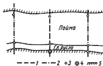
Рис.5.3. Примерная схема расположения уклонных постов на створах с широкими поймами 1 - гидроствор; 2 - створы уклонных постов; 3 - уклонный гидрологический пост; 4 - основной гидрологический пост; 5 - коренной берег
