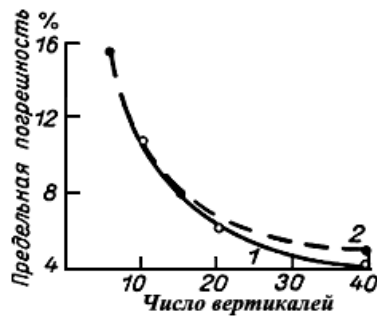
Рис.12.2. Зависимость предельной погрешности в измерении расхода воды 95%-ной обеспеченности от числа скоростных вертикалей 1 - по данным Р.Херши; 2 - по данным Н.К.Сибиряковой
