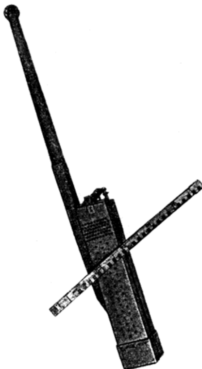
Рис.10.2. Шугобатометр ГР-3
