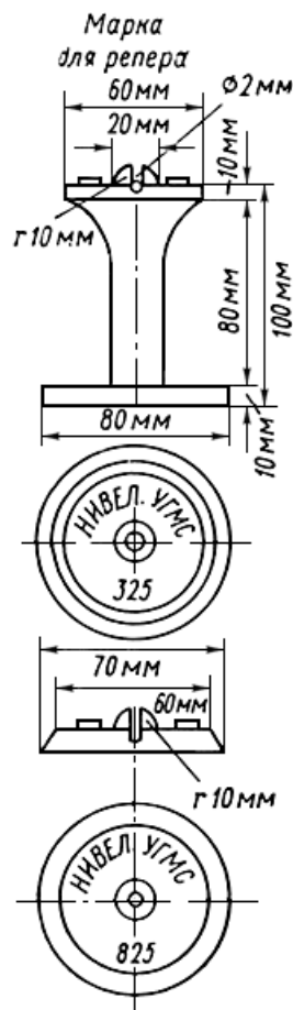
Рис.3. Марка для грунтовых и скальных реперов
