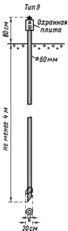
Рис.6. Грунтовый репер для районов подвижных песков
