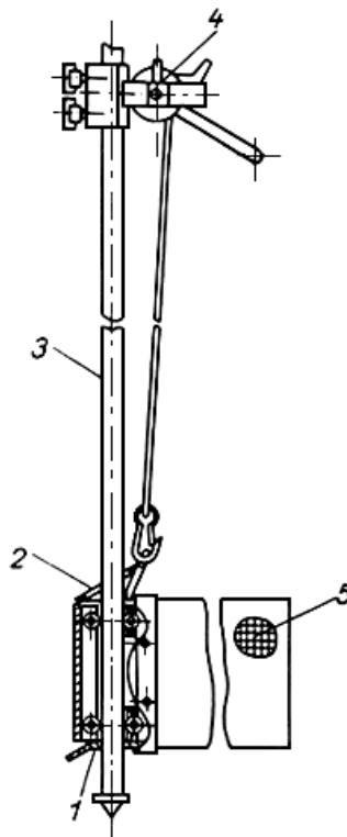
Рис.12.7. Батометр сетчатый ПИ-29 1 - рама; 2 - погружатель; 3 - штанга; 4 - лебедка; 5 - сетка
