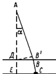
Рис.6.5. Схема измерения глубин при высоко подвешенном стальном канате
