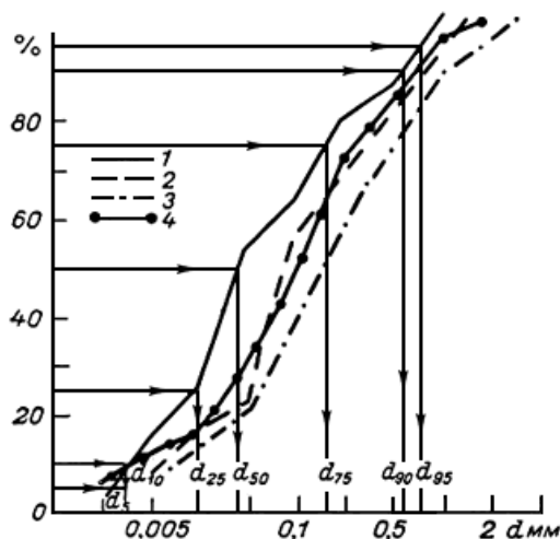
Рис.8.9. Интегральные кривые гранулометрического состава донных наносов (р.Песчаная - с.Заречное, 1975 г.)
