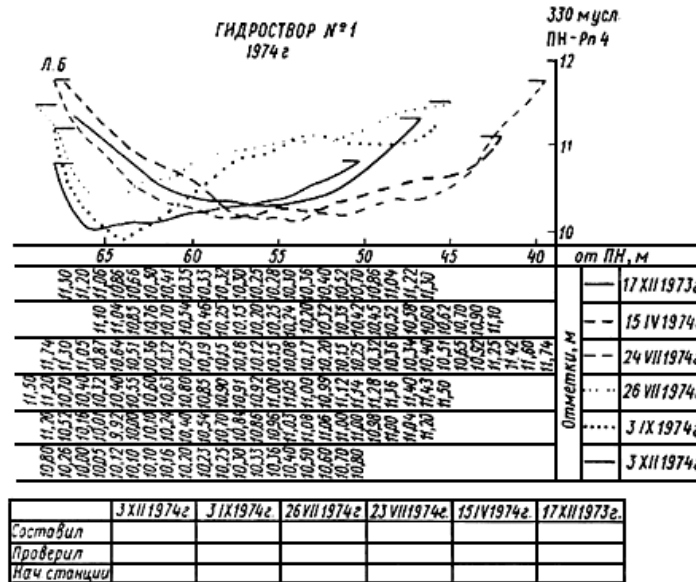
Рис.6.3. Совмещенные профили главного русла в гидростворе
