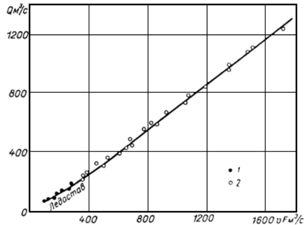
Рис.6.6. График зависимости Q = f(v_{0,2}F) 1 - при ледоставе; 2 - при открытом русле
