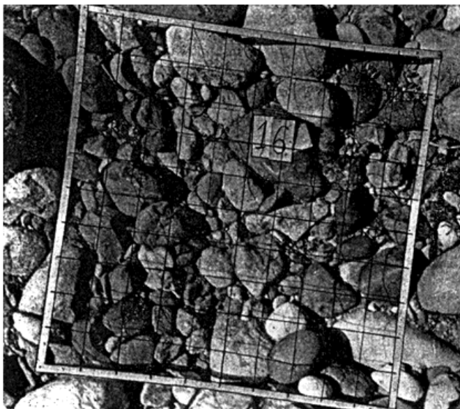
Рис.8.2. Фотография крупных донных наносов (р.Картан - с.В.Картан, N 16)
