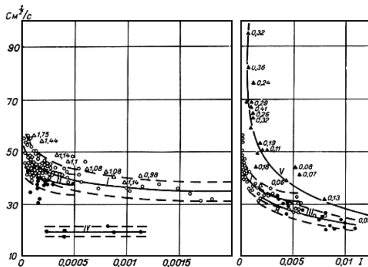
Рис.5.5. Зависимости коэффициента C формулы Шези от уклона водной поверхности. Цифры у точек - коэффициенты устойчивости русел Лохтина, пунктир - границы 10%-ных отклонений
