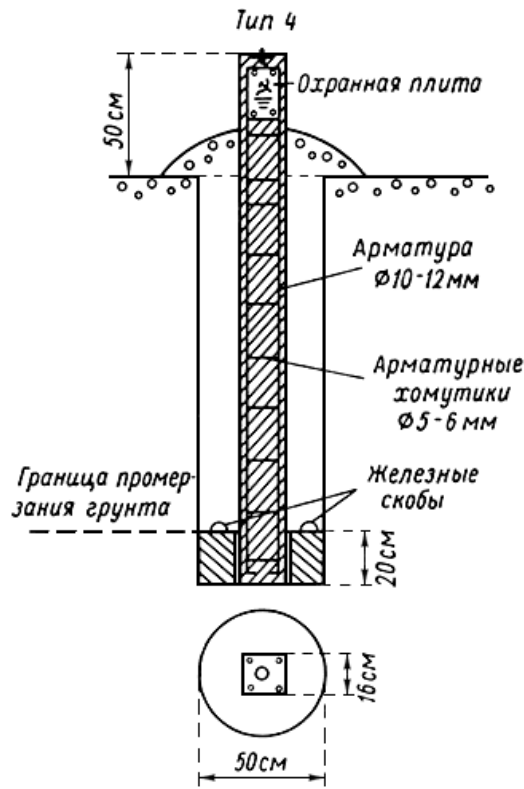
Рис.2. Грунтовый репер нивелирования III и IV классов для южной зоны сезонного промерзания грунтов
