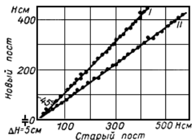
Рис.4.1. График связи уровней старого и нового постов
