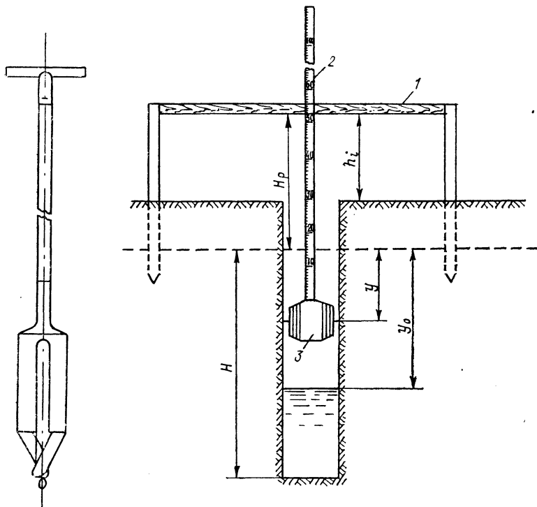
Рис. 23.5. Бур Розанова.
