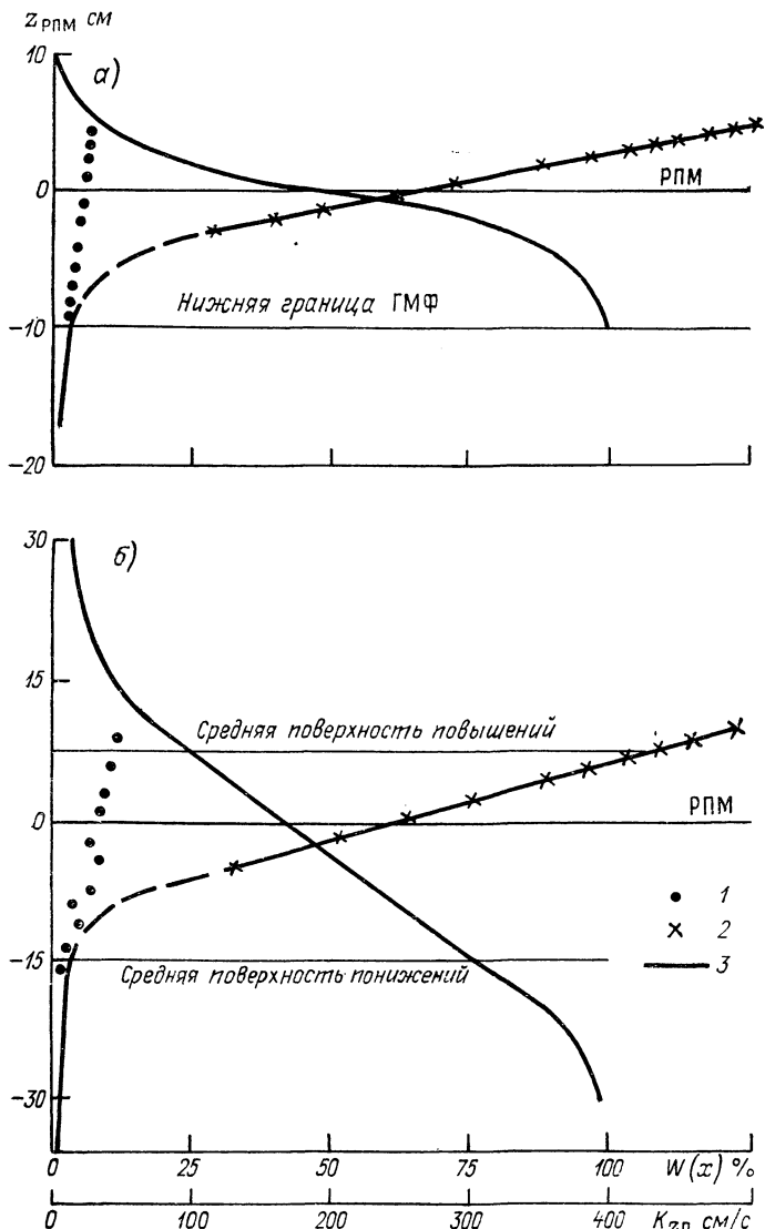
Рис. 23.4. Совмещение кривых K_{z_{cp}} = f(z) (1), K_{z_{п}} = f(z) (2) и W(x) (3) для мохово-травяных (а) и лесных и облесенных (б) микроландшафтов.
