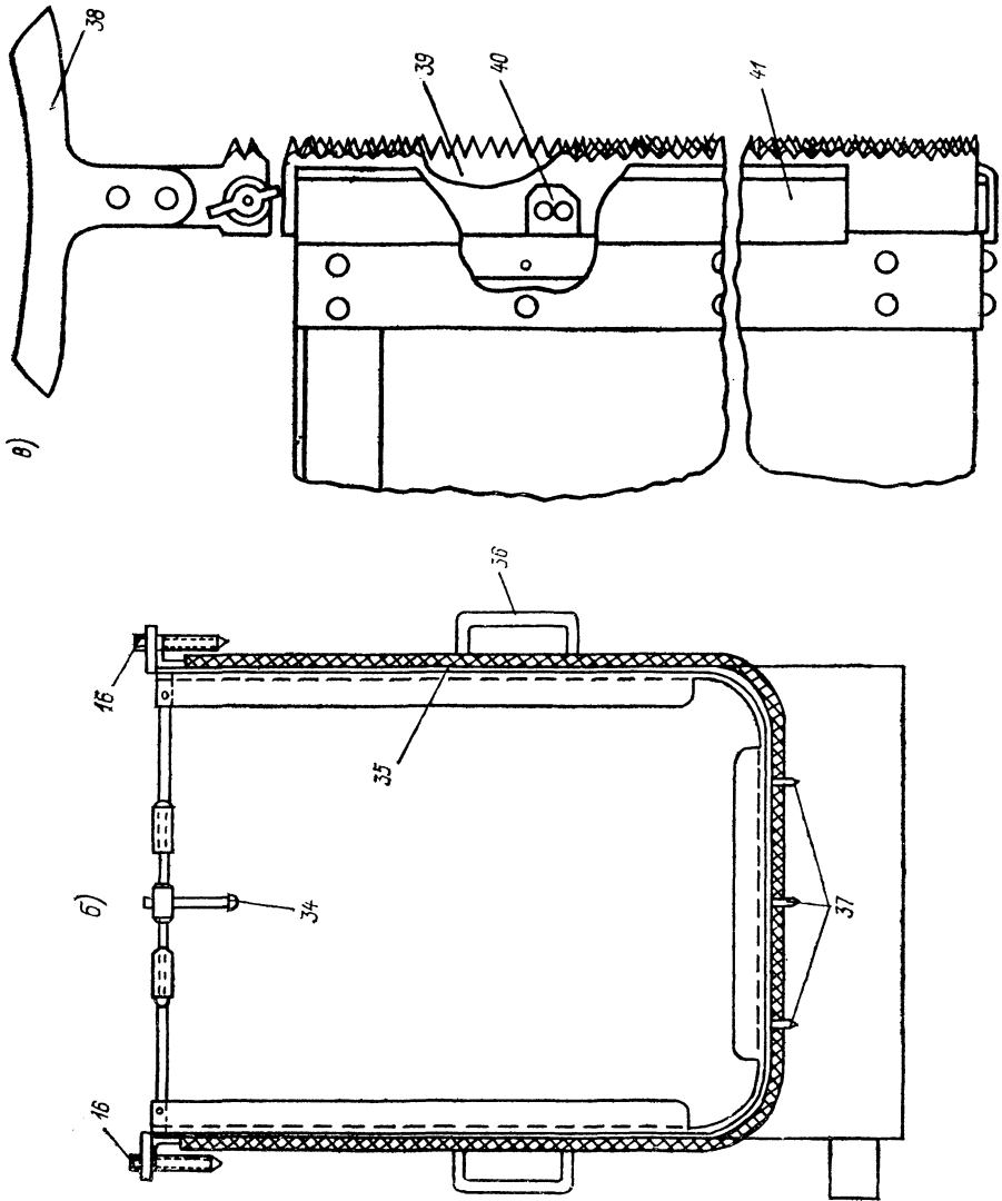
Рис. 23.1. Комплект фильтрационного оборудо- дования (а), торцевая часть фильтрационного отсека в месте его соеди- нения с верхним отсеком (б) и крепление подвиж- ной пилы (в).
