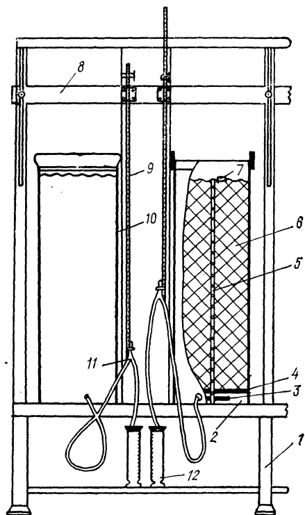
Рис. 26.1. Схема установки для определения водоотдачи методом дренирования колонн торфа.
