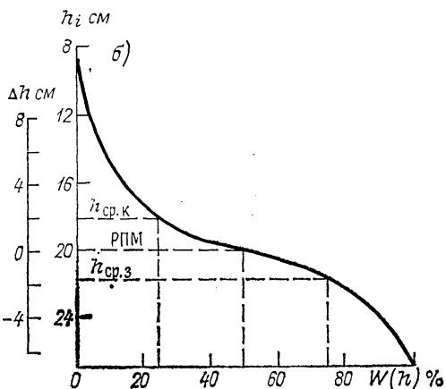
Рис. 15.1. Схема определения по интегральной кривой распределения высот микрорельефа W(h_i) значений F_t (а) и средних высот относительно РПБ повышений ( h_{ср.к} ) и понижений ( h_{ср.з} ) ГФМ (б).
