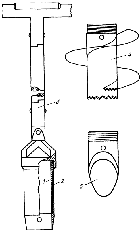
Рис. 14.1. Проботборник со сменными резцами.
