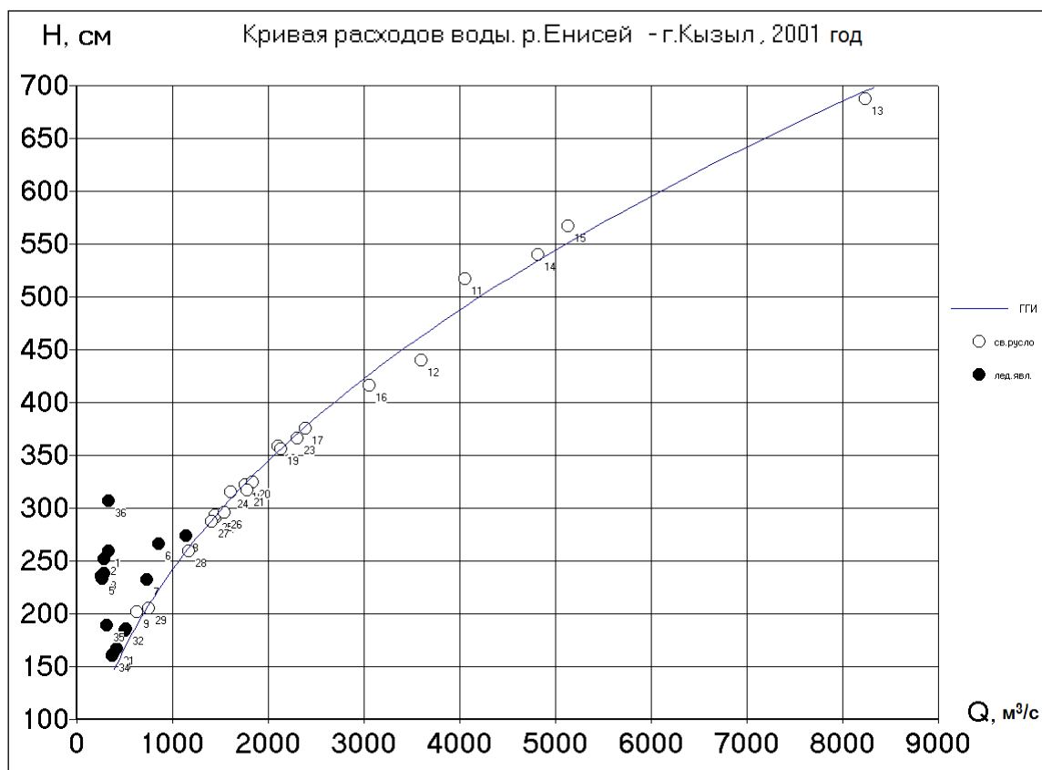
Рисунок А.1 – Зависимость расходов воды от уровней
