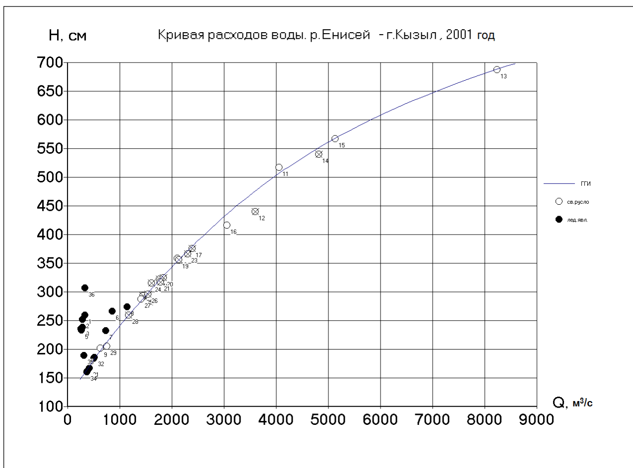
Рисунок А.2 – Зависимость расходов воды от уровней, полученная по сокращенной совокупности из 10 ИПВ
